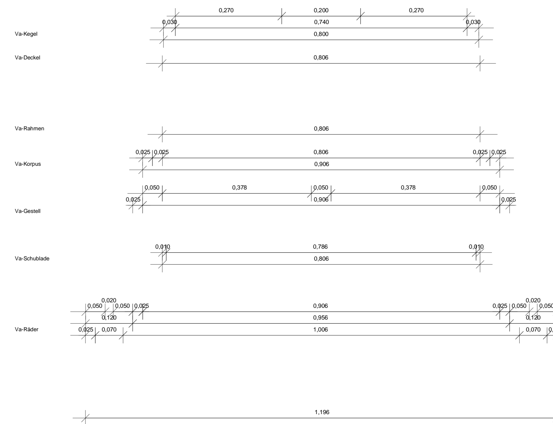
ENTWURF KELLNERWAGEN M 1:5 ANSICHT GRIFFE Restaurant Kleines Steakhaus Herr Sascha Salcin SH-HS-01.14 23.01.14 1-001-02 ARCHITEXTURBÜRO DIPL.-ING. MICHAEL DÖRSTELMANN
