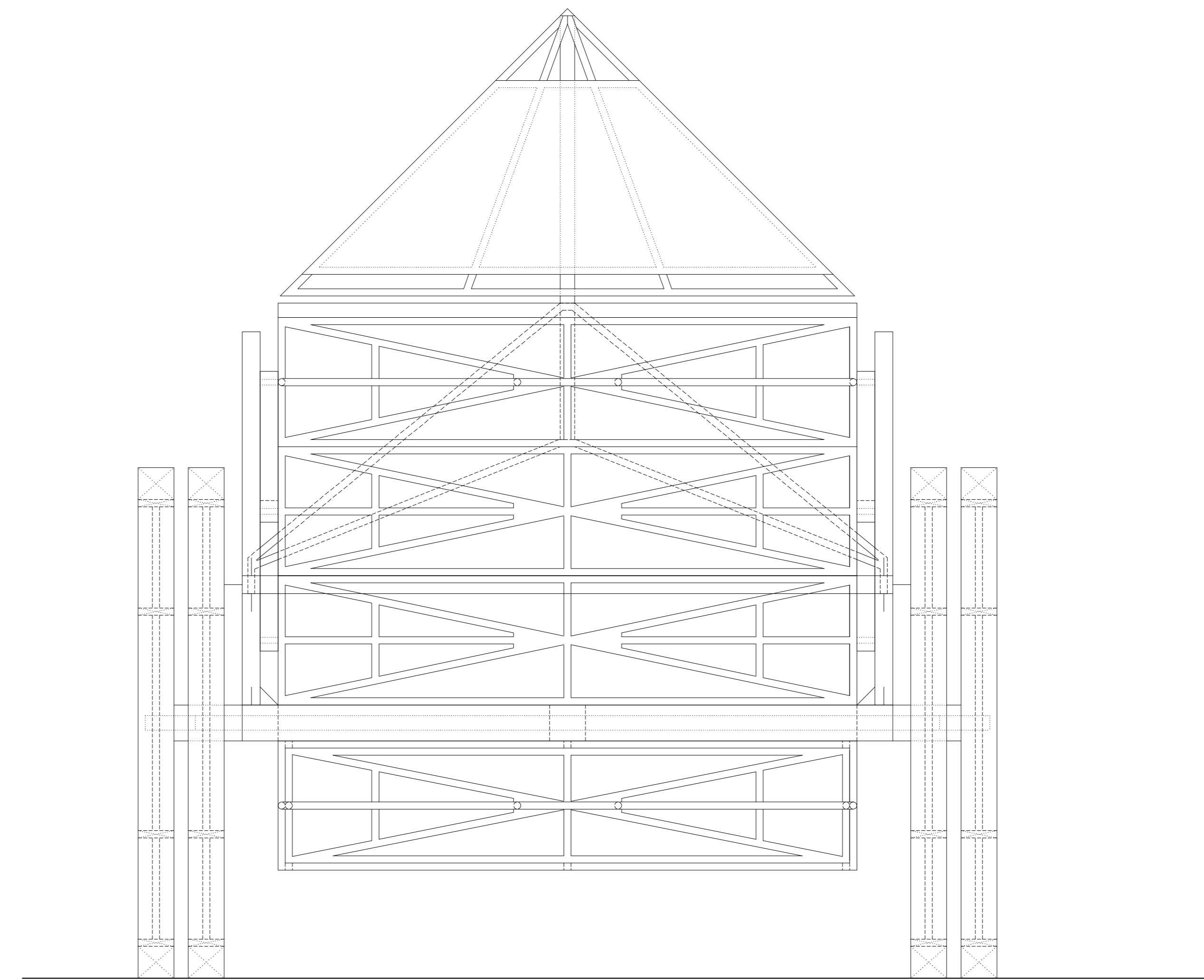
ENTWURF KELLNERWAGEN M 1:5 ANSICHT GRIFFE Restaurant Kleines Steakhaus Herr Sascha Salcin SH-HS-01.14 23.01.14 1-001-02 ARCHITEXTURBÜRO DIPL.-ING. MICHAEL DÖRSTELMANN
